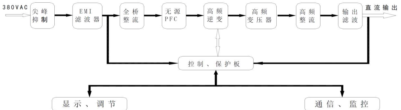
图1 高频开关电源模块原理框图
