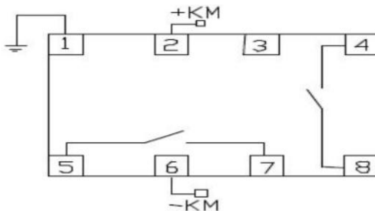
图2-3-5 绝缘监测
