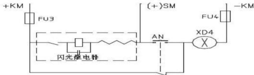
图2-3-4 闪光回路
